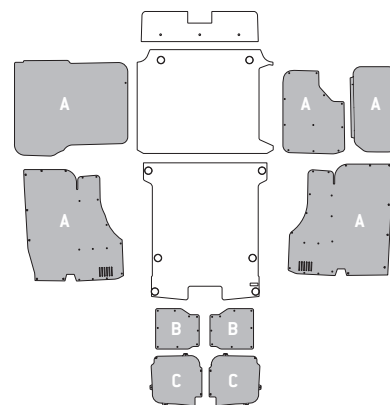
Modelo - Model long (L2)
